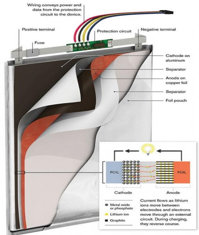
Figure 4 : Principaux constituants d'un élément Lithium-ion
