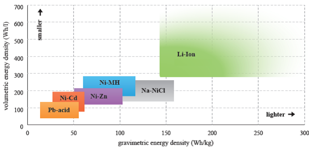
Figure 1 : Densité d'énergie massique et volumique des principales technologies commerciales
