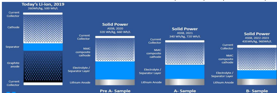
Figure 7 : Construction d'un élément Lithium tout solide - Source Solid Power, 2020
