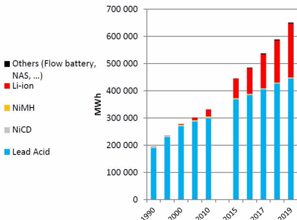
Figure 2 : Evolution du marché mondial des batteries rechargeables de 1990 à aujourd'hui, toutes applications confondues. Source Avicenne Consulting, 2020
