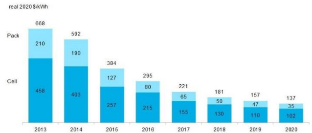
Figure 3 : Evolution du prix des éléments et batteries Li-ion 2013-2020 - Source Bloomberg NEF, 2020
