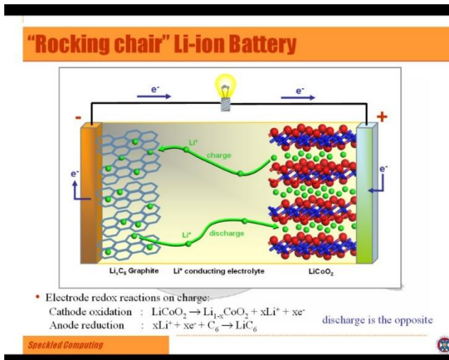
Figure 5 : Principe de fonctionnement d'un élément Lithium-ion
